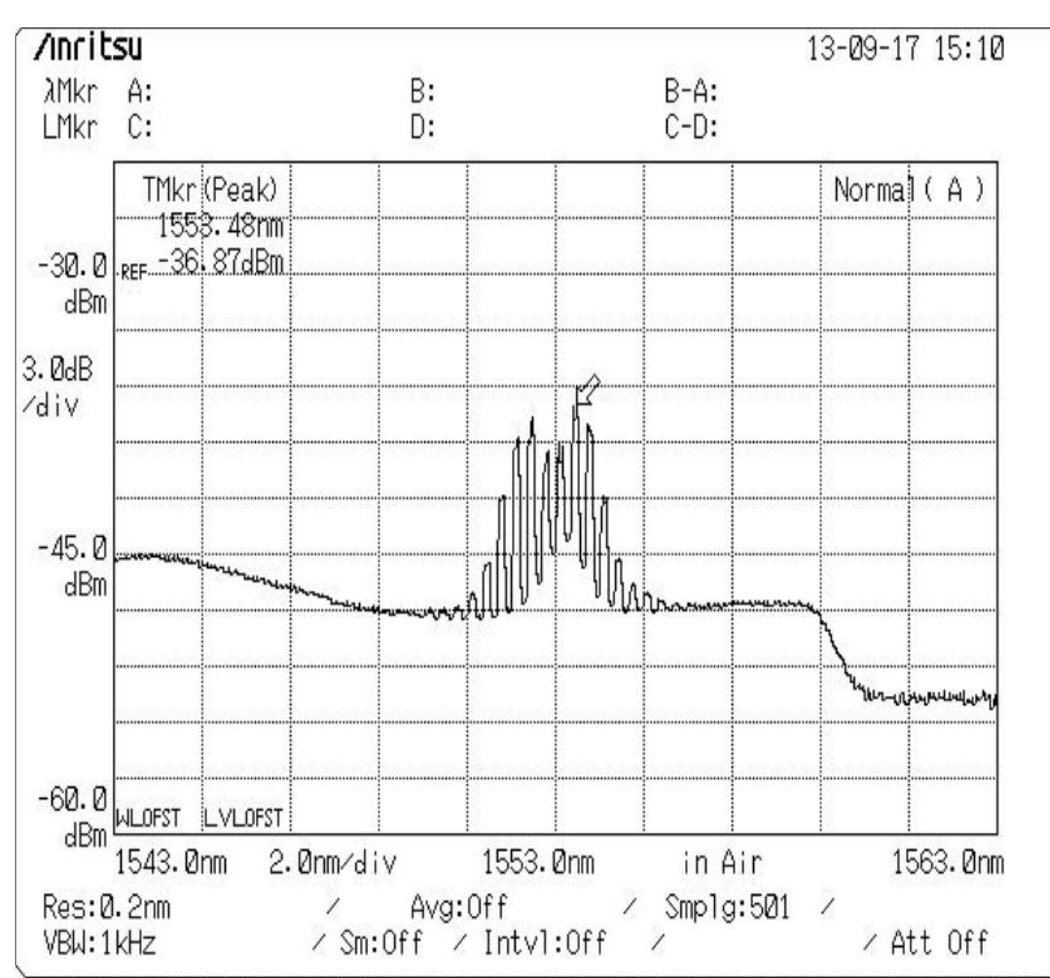
图 2. 峰值光功率 1 kW (1ns) 光谱图
