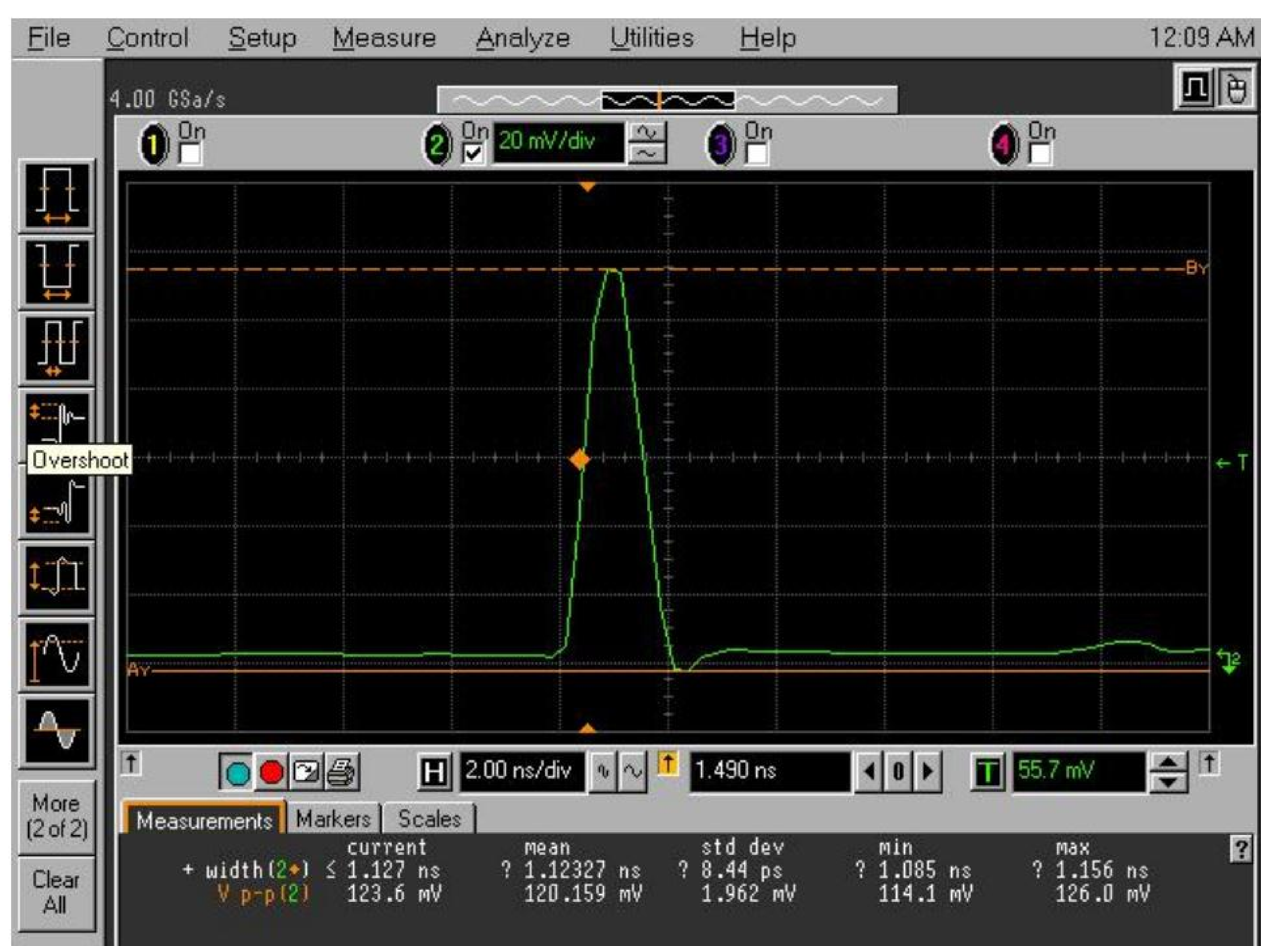
图 1. 峰值光功率 1 kW (1ns) 单脉冲波形图
