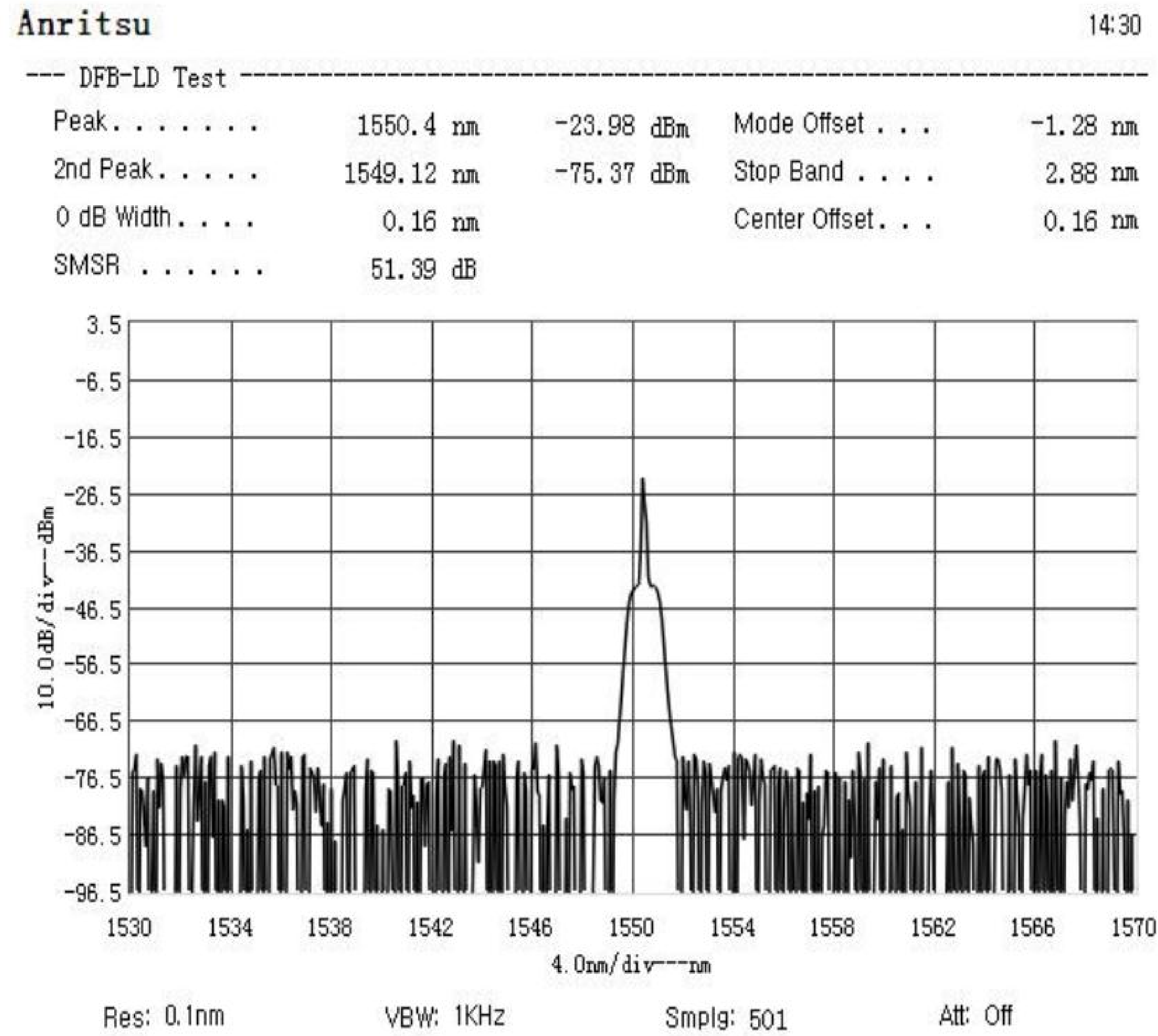
50W-5ns-10KHz
