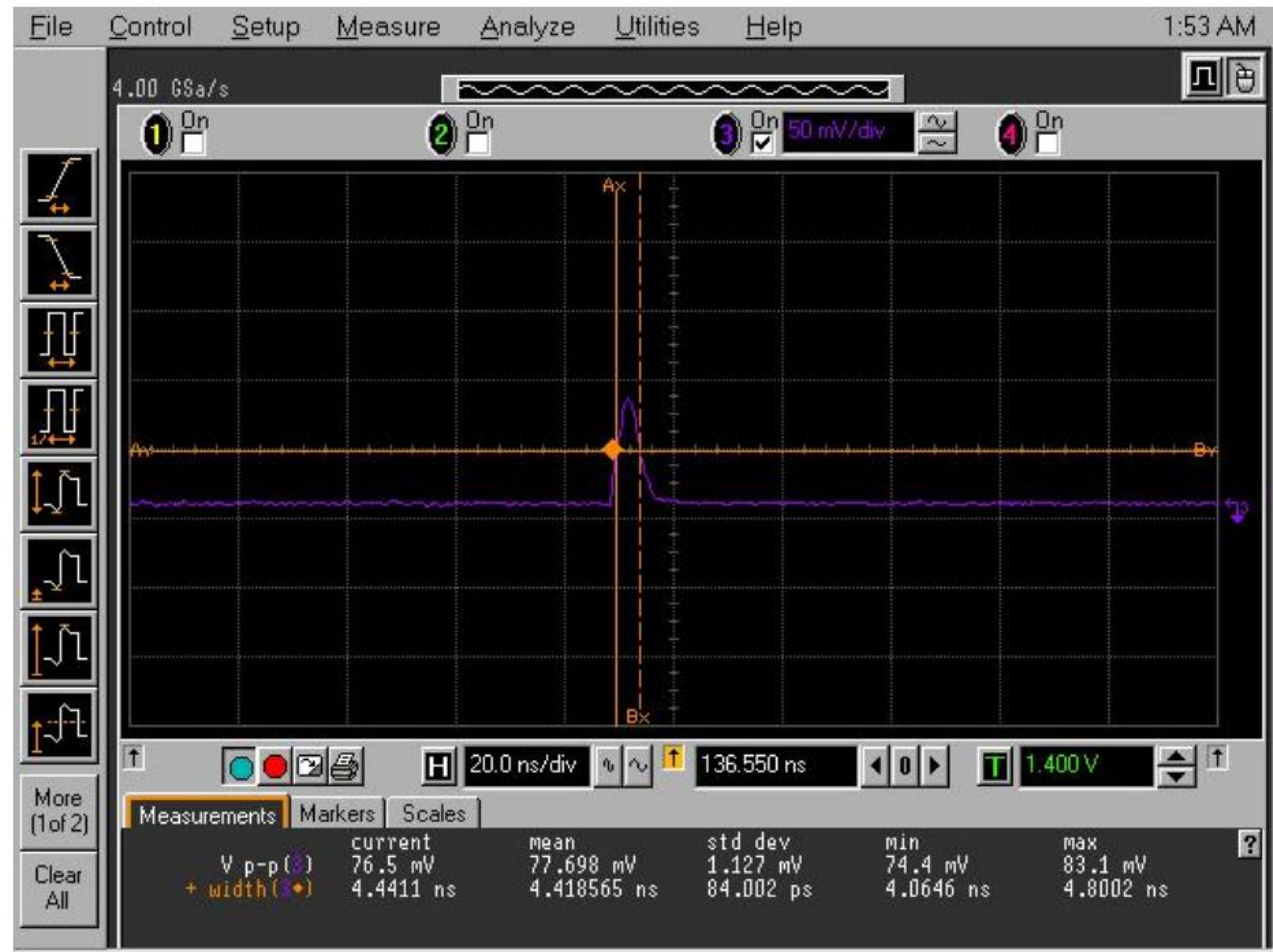
50W-5ns-5KHz
